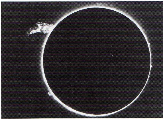
彩層と吹き上がるプロミネンス
