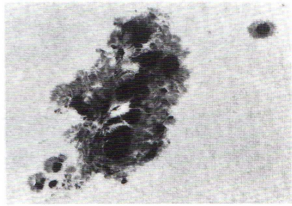
太陽黒点の例
